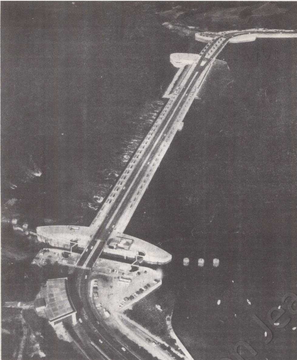
L'usine marémotrice de la Rance.
